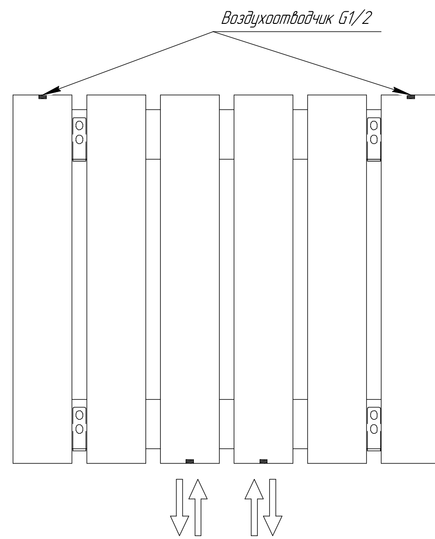
Подключение нижнее "динаклем" 0100
