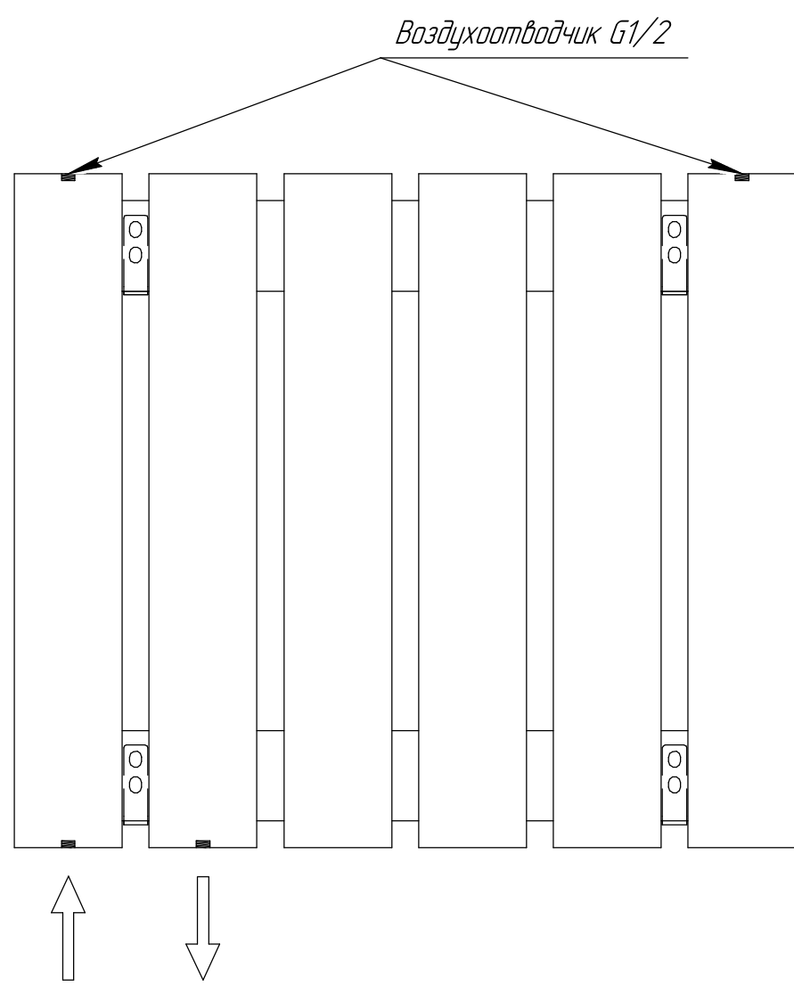
Подключение нижнее "динаклем" 1100
