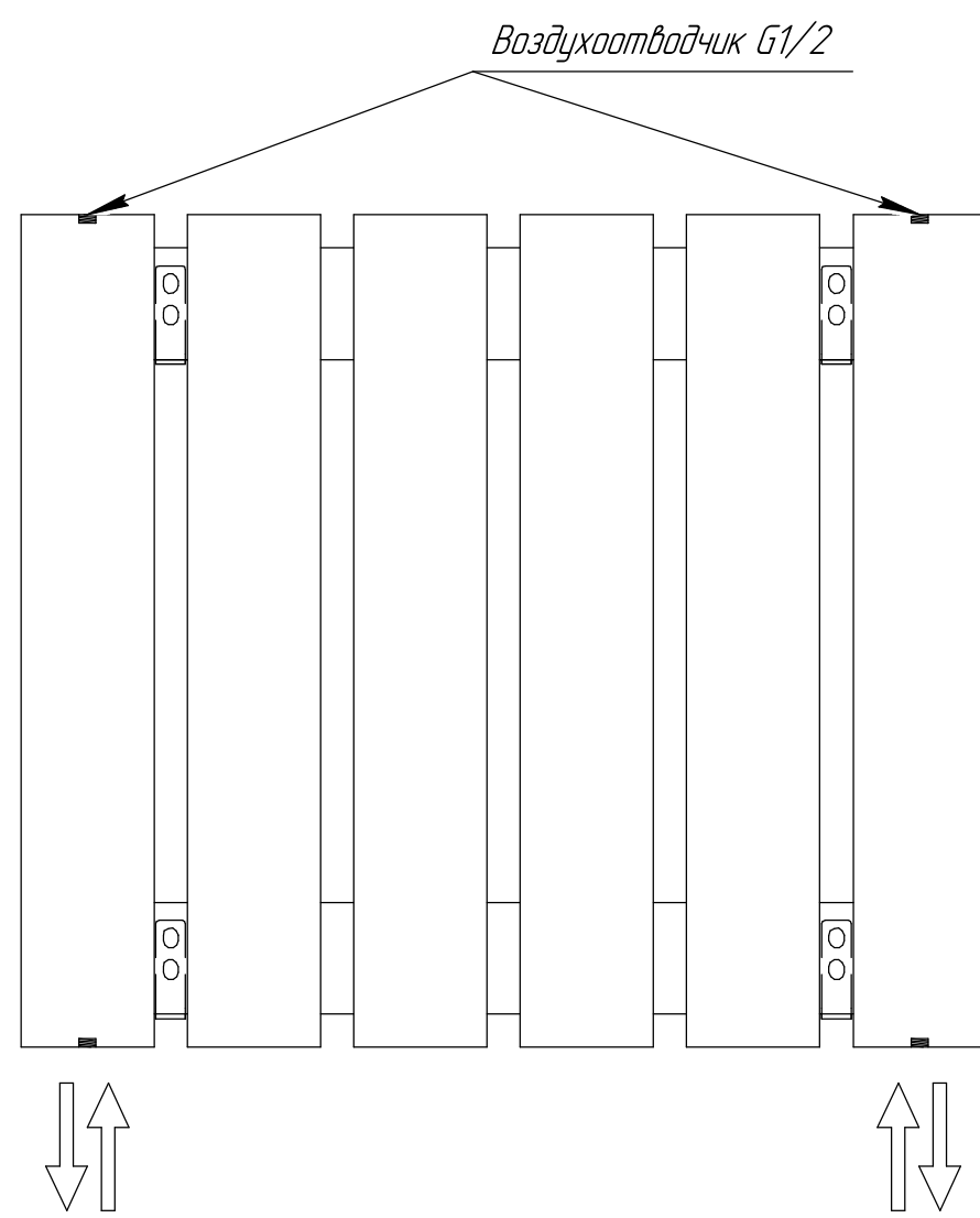
Подключение нижнее разнесенное 117
